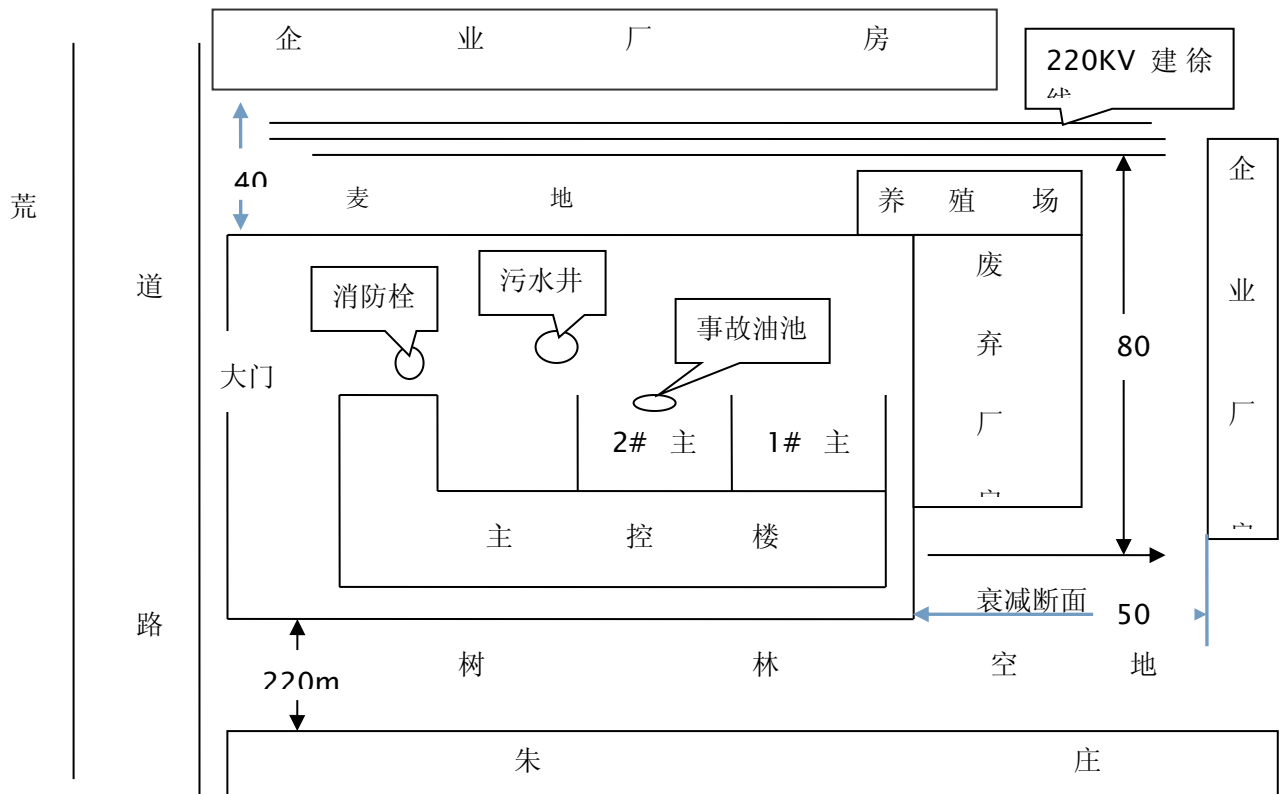
图强变电站平面示意图
