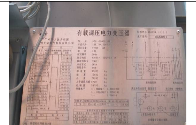
主变铭牌
