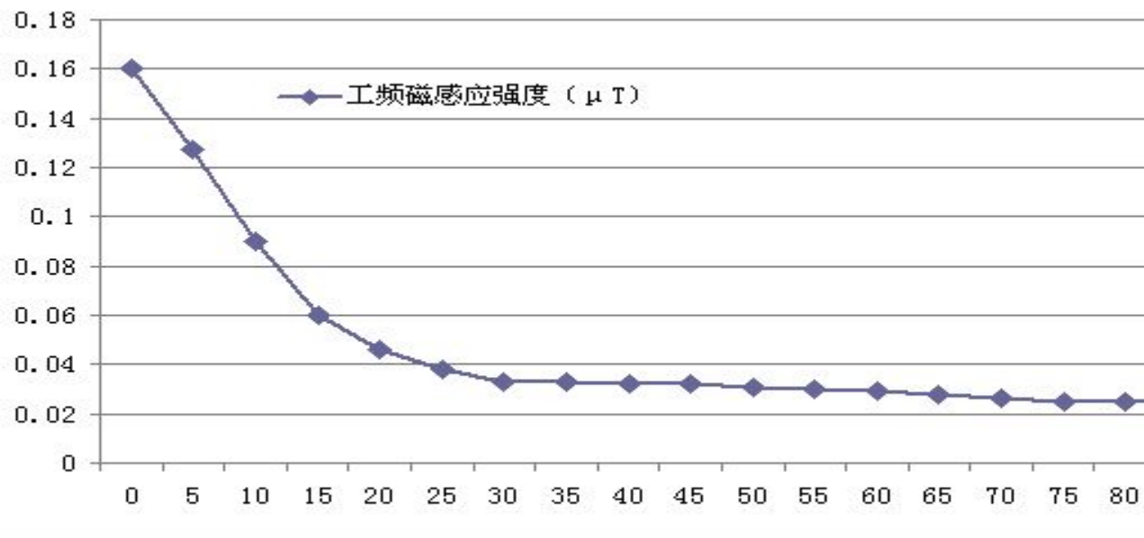
图 8-2 长乐（新城）输变电工程线路衰减断面工频磁场衰减情况
